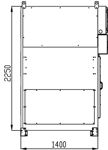
YANDAN GÖRÜNÜŞ LATERAL VIEW
